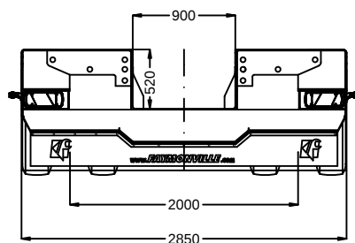
Heckansicht / rear view
